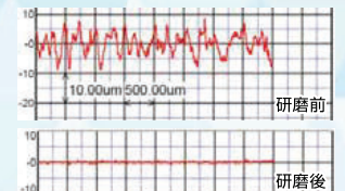
研磨前後の表面粗さ測定
